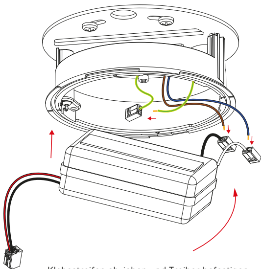
Klebestreifen abziehen und Treiber befestigen
