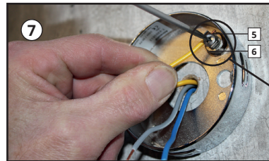
Item-No: [5] PFL-264 [6] PFL-263
